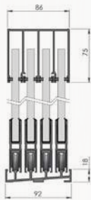
Afmetingen 4-sporige rails, verkrijgbaar in de lengtes: 2900, 3900, 4900 en 5900mm.
